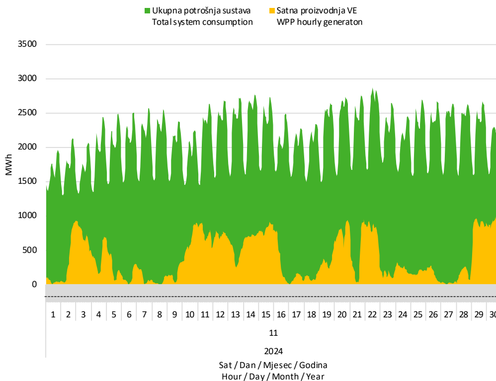
Slika 7 Usporedba satnog dijagrama opterećenja sustava i proizvodnje vjetroelektrana u studenom 2024. godine
