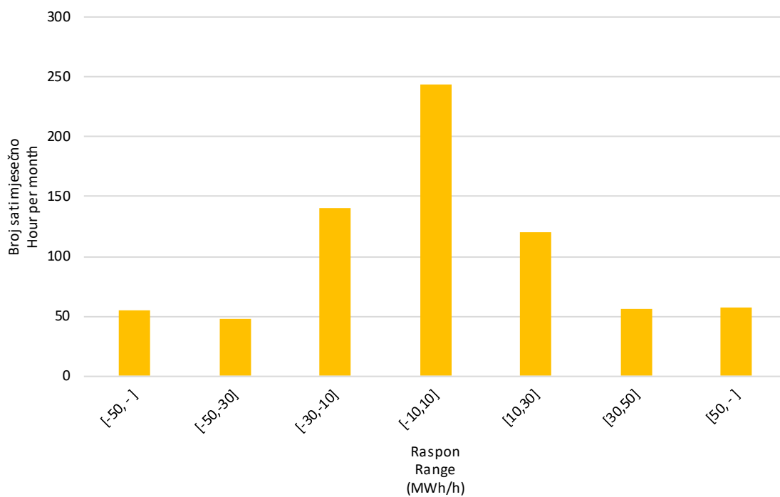
Slika 10 Statistička raspodjela satnih promjena proizvodnje VE u studenom 2024. godine
