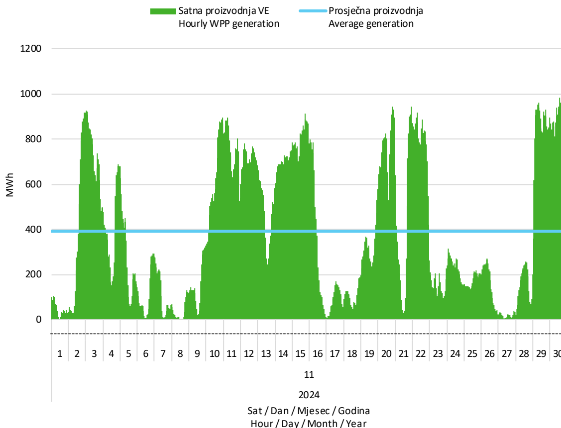
Slika 2 Satna proizvodnja svih vjetroelektrana u studenom 2024. godine
