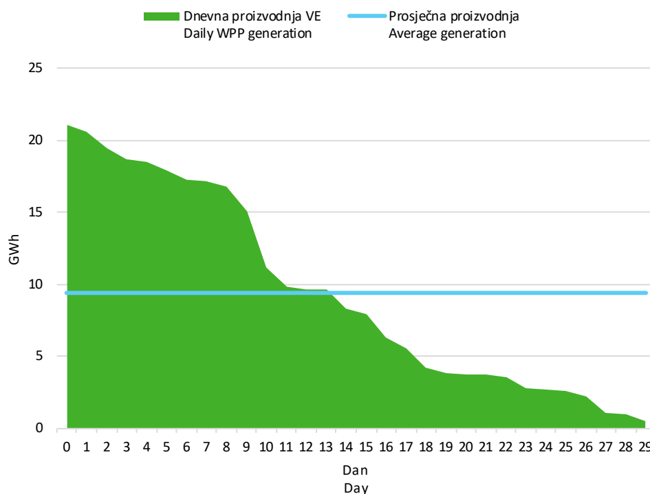
Slika 6 Krivulja trajanja dnevne proizvodnje vjetroelektrana u studenom 2024. godine
