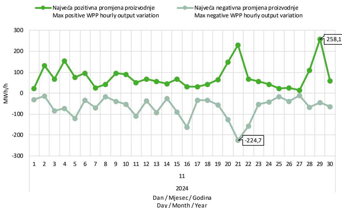
Slika 9 Maksimalna pozitivna i maksimalna negativna promjena satne proizvodnje VE u studenom 2024. godine
