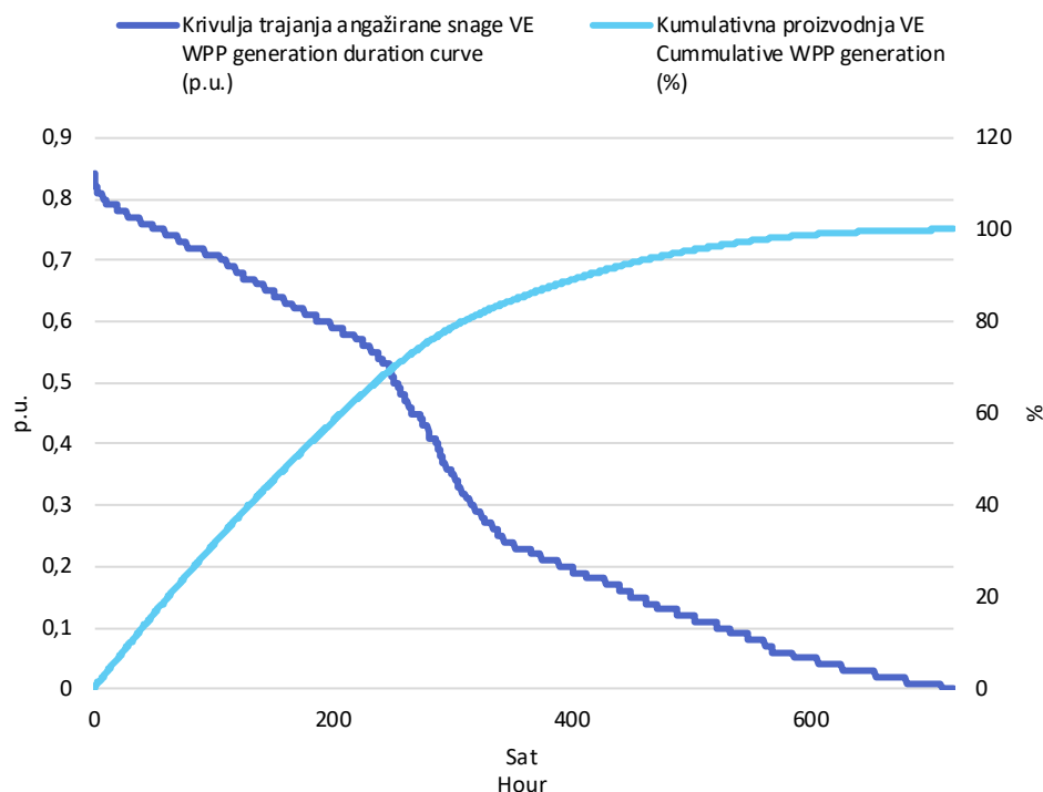
Slika 3 Krivulja trajanja angažirane snage svih VE i kumulativna proizvodnja VE u studenom 2024. godine u jediničnim vrijednostima
