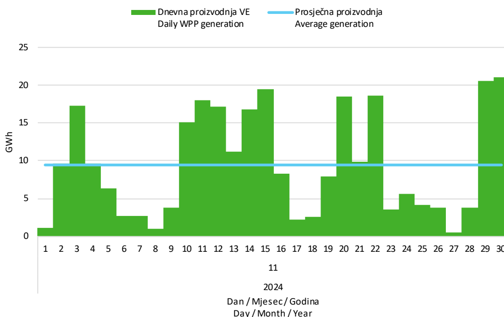
Slika 5 Dnevna proizvodnja svih vjetroelektrana u studenom 2024. godine
