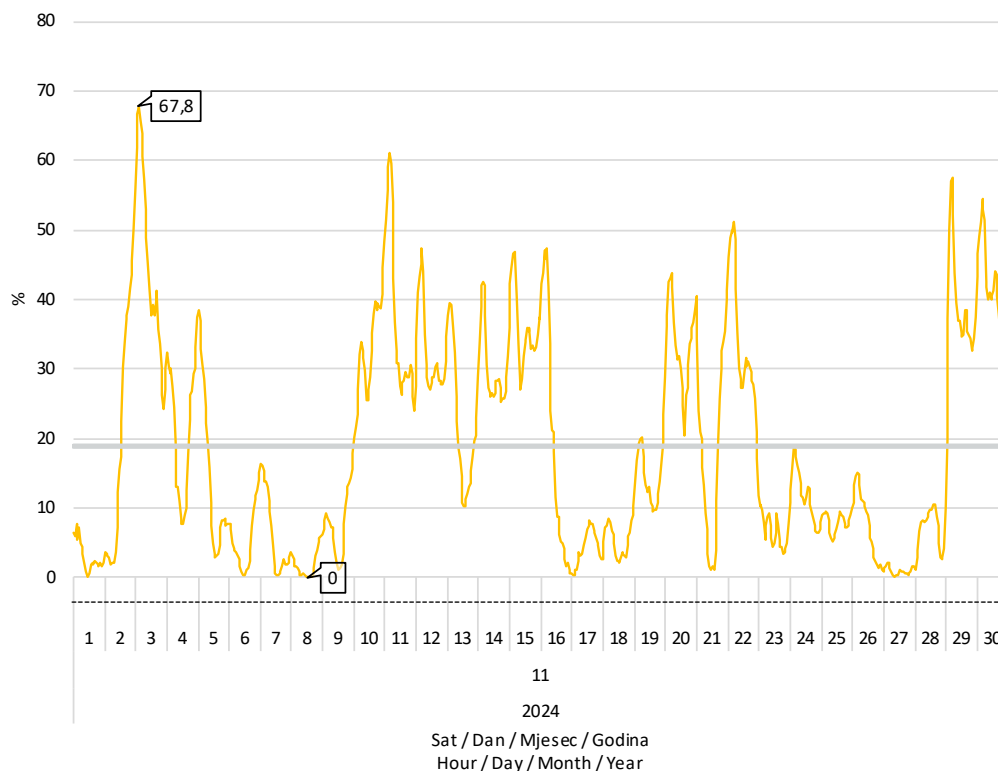
Slika 8 Udio proizvodnje vjetroelektrana u pokrivanju satnog opterećenja elektroenergetskog sustava u studenom 2024. godine
